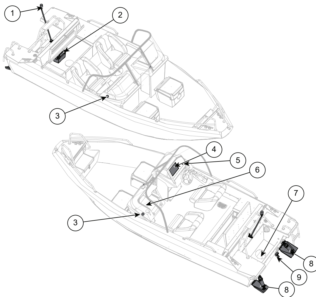
Abbildung 8.2 Buster X Elektrische Ausrüstung
