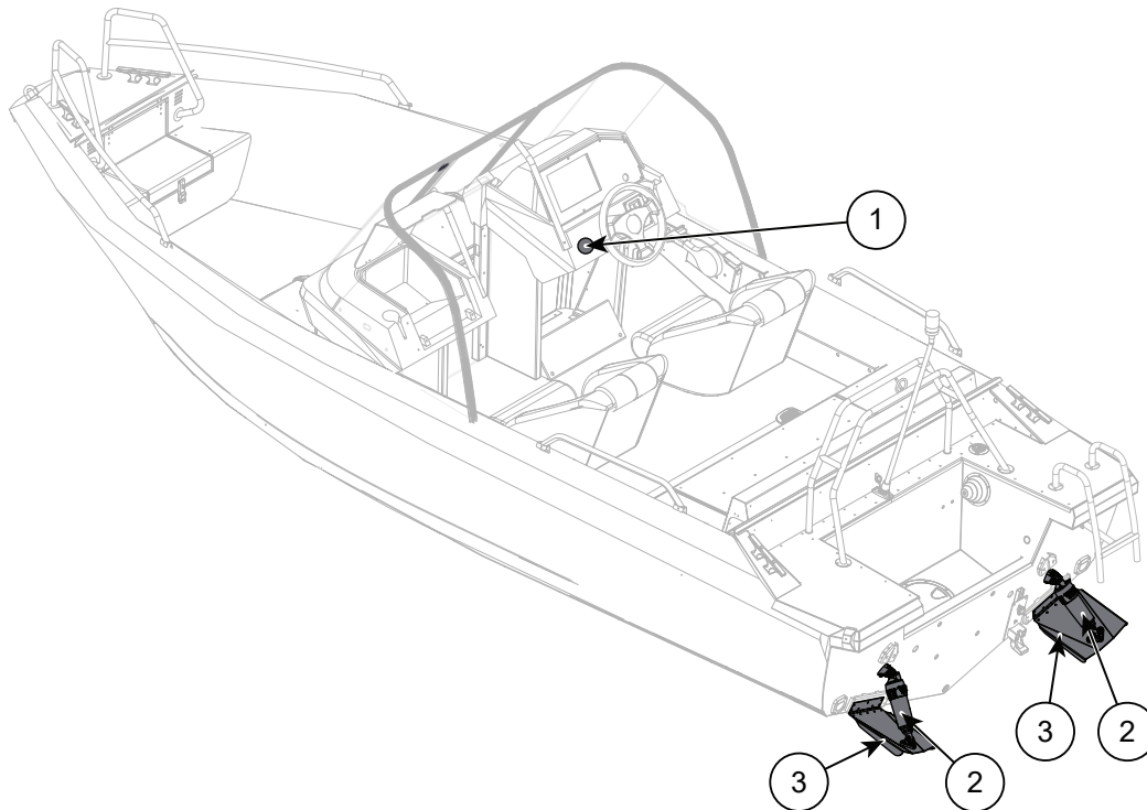
Abbildung 5.4 Komponenten des Trimmsystems Buster X
