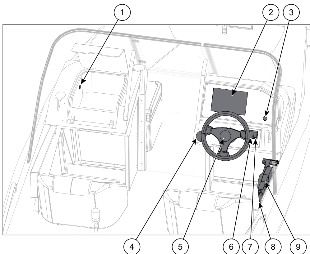
Abbildung 5.1 Buster X Bedienelemente am Steuerstand
