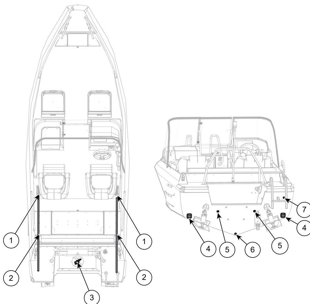
Abbildung 9.1 Buster X Entwässerungsgeräte
