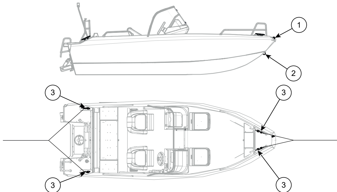
Abbildung 5.5 Buster X Befestigungs- und Schlepppunkte
